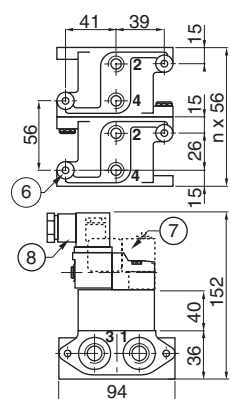
клапан 261
