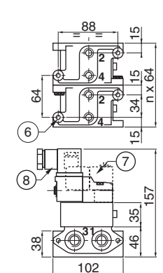
клапан 262
